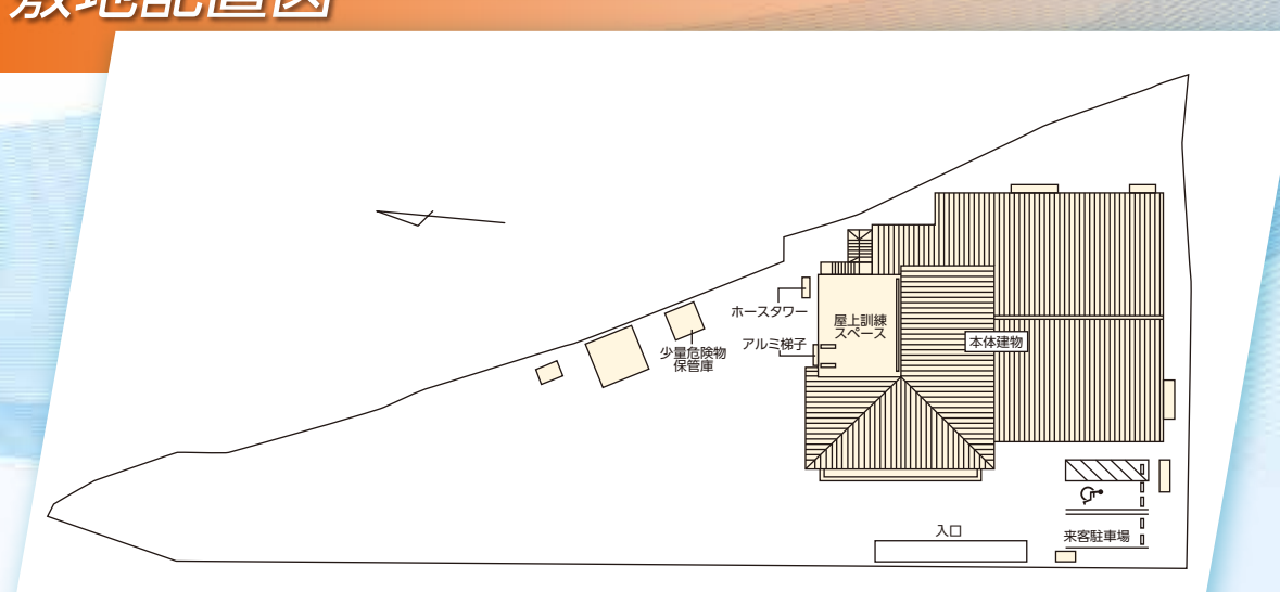
敷地配置図
